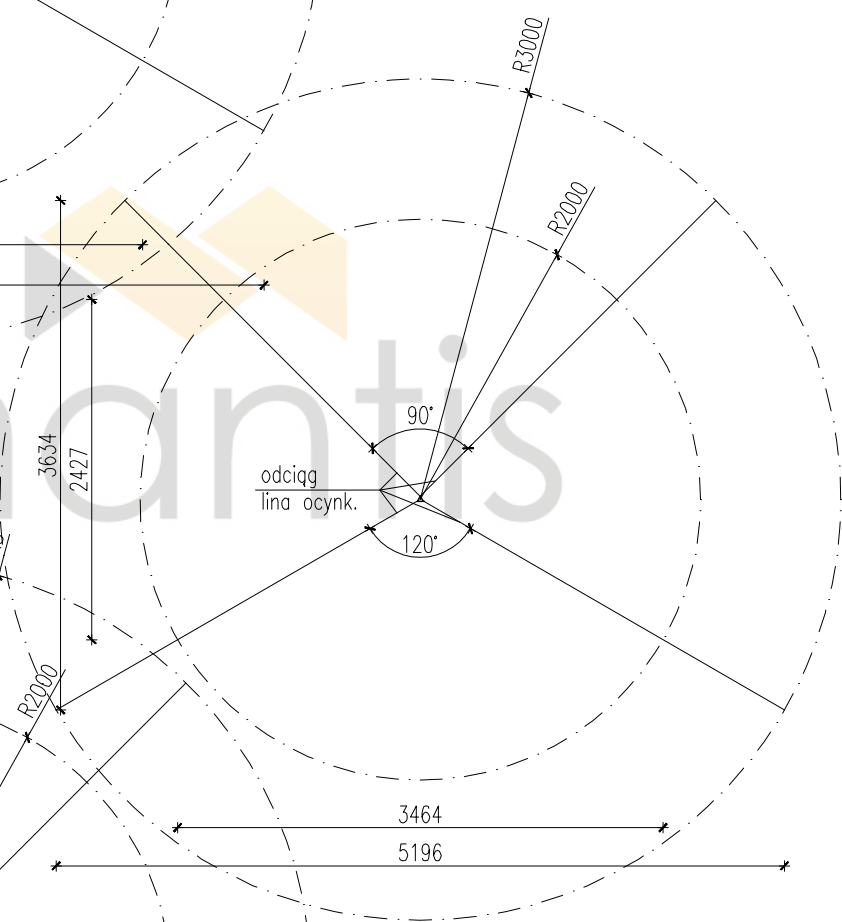
RZUT ODCIĄGÓW (wymiary w cm) -SKALA 1:500 WARIANT Z 4 ODCIĄGAMI
