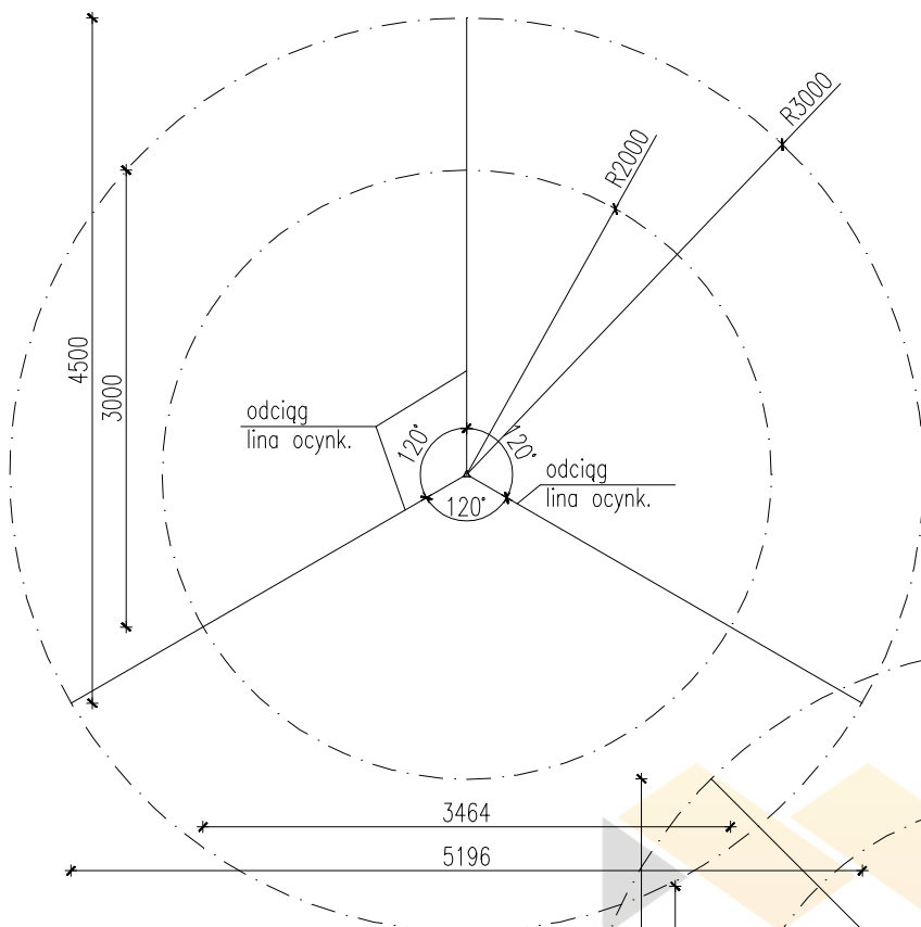
RZUT ODCIĄGÓW (wymiary w cm) -SKALA 1:500 WARIANT Z 3 ODCIĄGAMI
