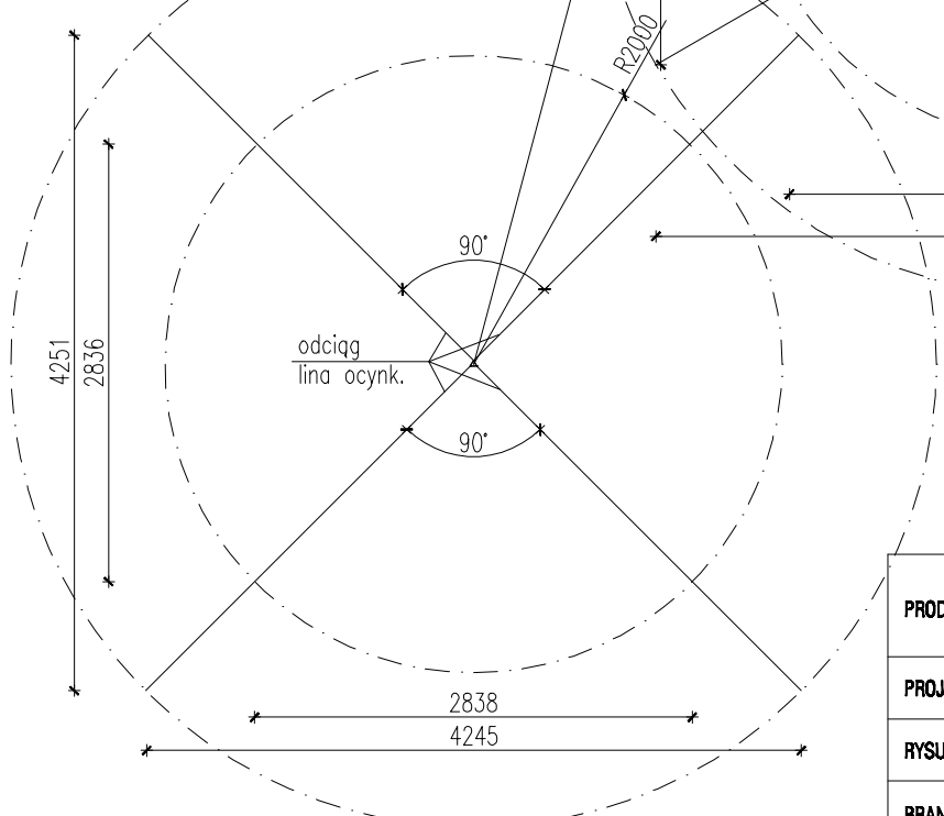
RZUT ODCIĄGÓW (wymiary w cm) -SKALA 1:500 WARIANT Z 4 ODCIĄGAMI
