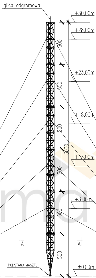
WIDOK PIONOWY, SKALA 1:200 (wymiary w cm)
