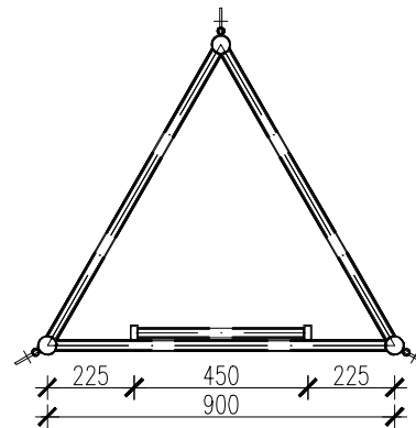
PRZEKRÓJ A-A, SKALA 1:20 (wymiały w mm)
