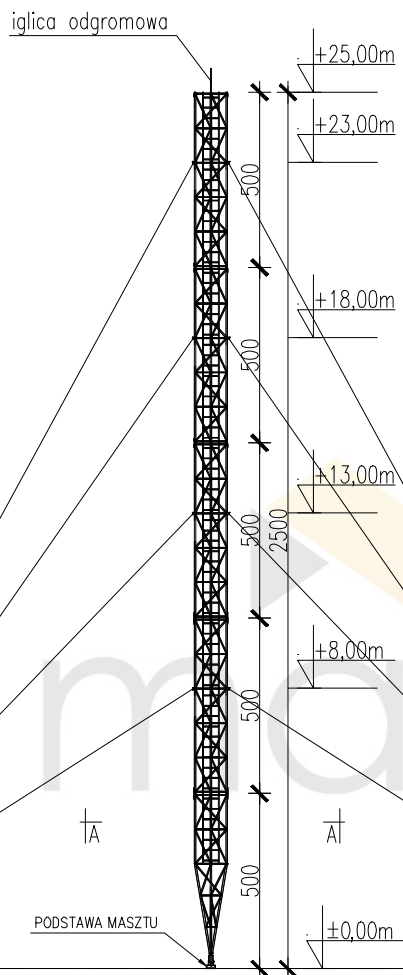
WIDOK PIONOWY, SKALA 1:200 (wymiały w cm)
