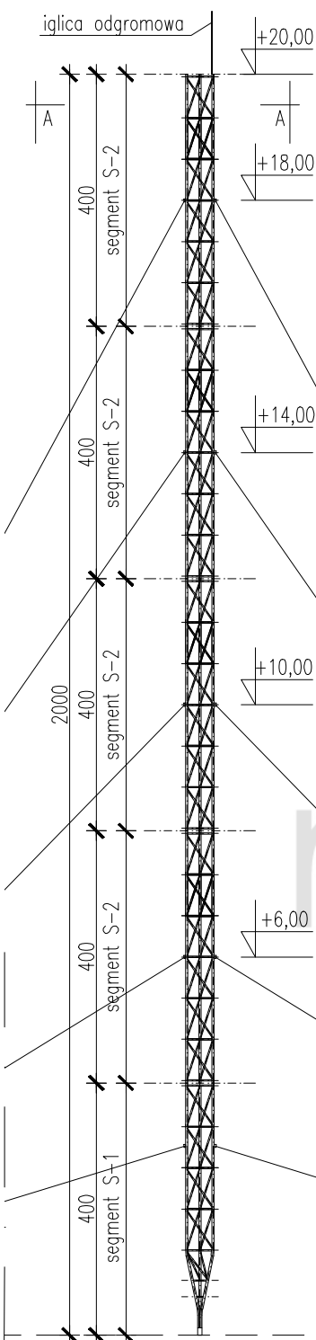
WIDOK PIONOWY, SKALA 1:100 (wymiar w cm)
